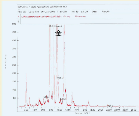
第32次出土帯執金具の表面拡大写真と成分分析データ
