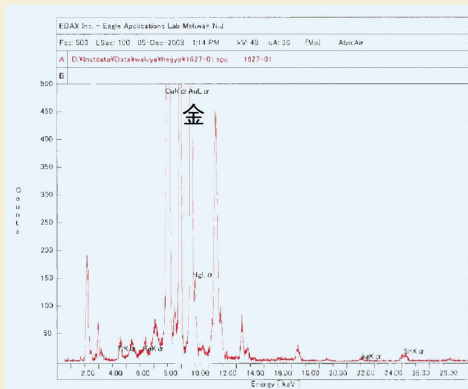
西大寺出土帯執金具の表面拡大写真と成分分析データ
