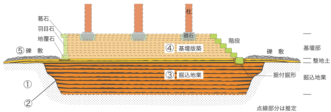
南門断面模式図
