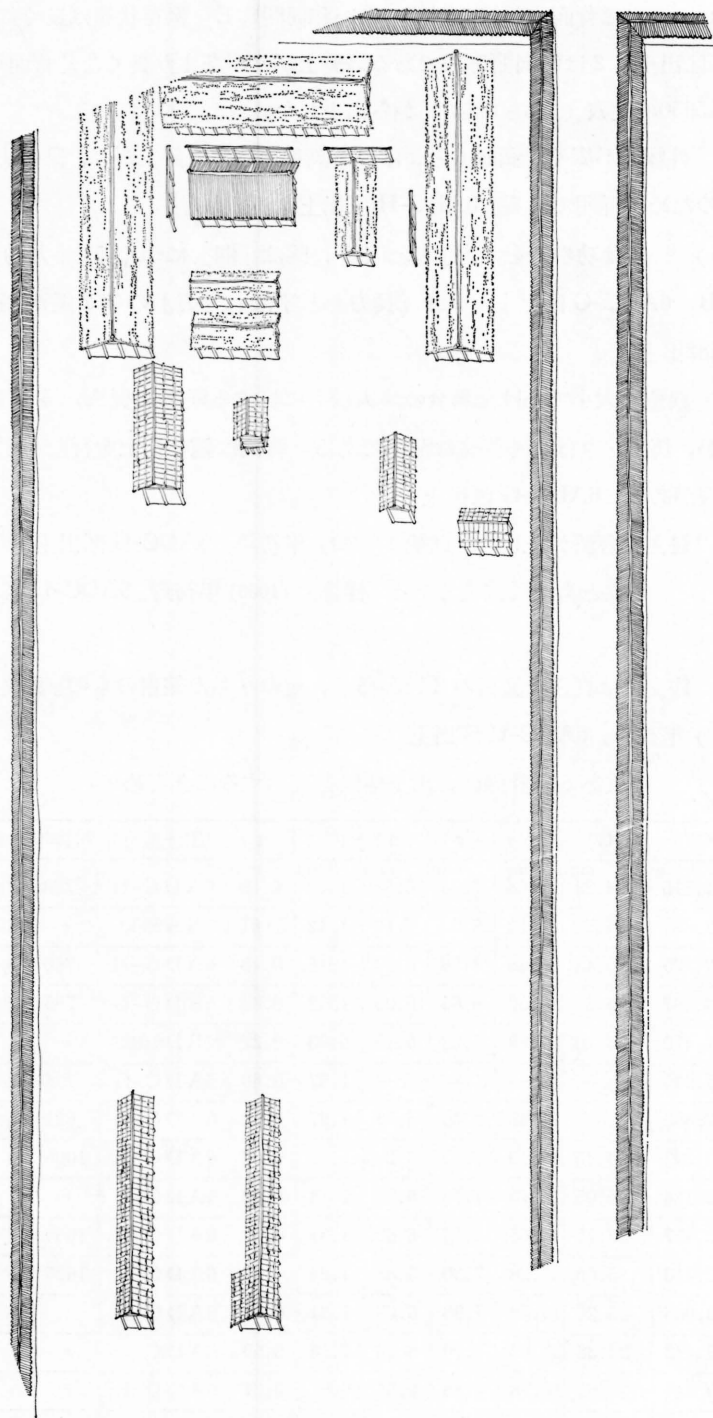
馬寮第IV期の遺構の想定図
