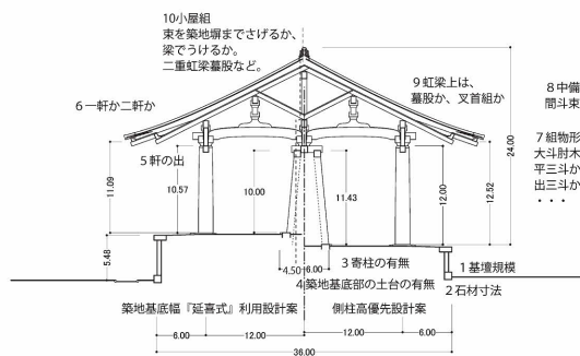
図56 築地回廊梁行標準断面案
