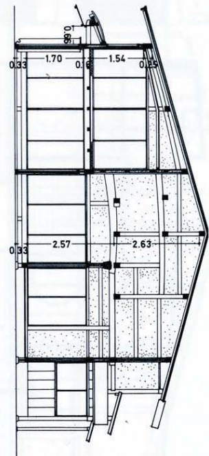
16-d 断面図
