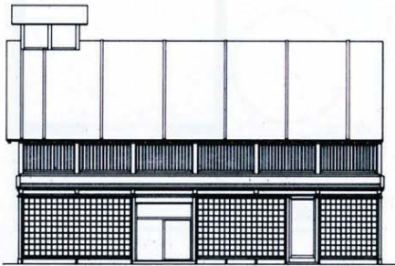
18-a 正面図
