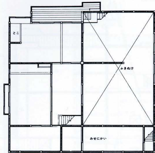
23-a 2階平面図
