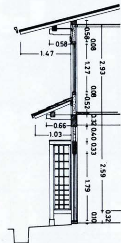
27-b 矩計図
