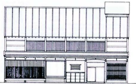
21-c 正面図
