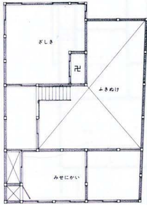
15-a 2階平面図
