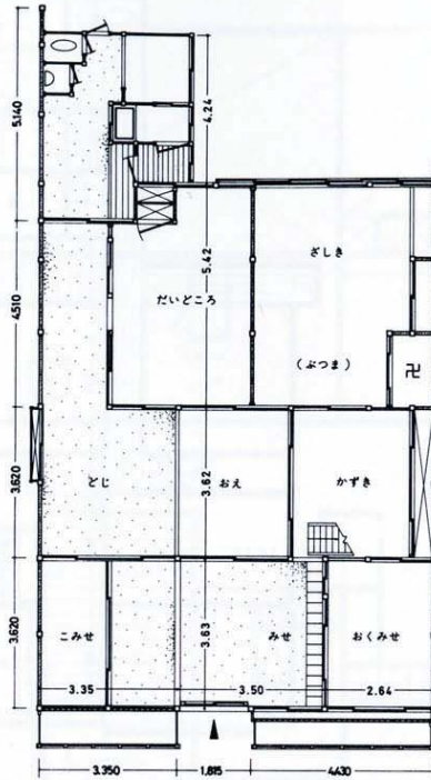
17-b 1階平面図
