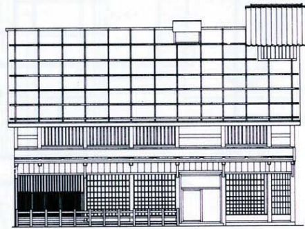
28-c 正面図
