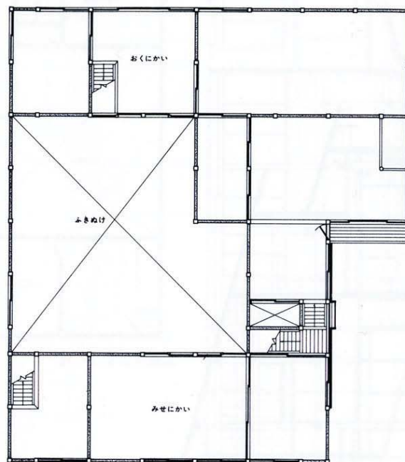
24-b 2階平面図
