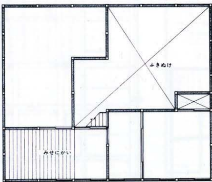
16-a 2階平面図
