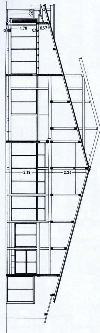
26-c 断面図
