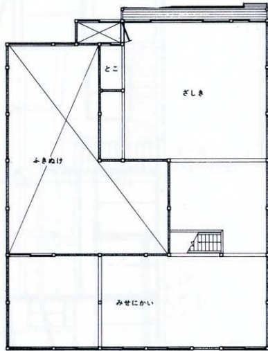
17-a 2階平面図
