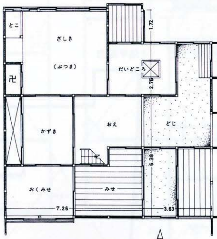
16-b 1階平面図
