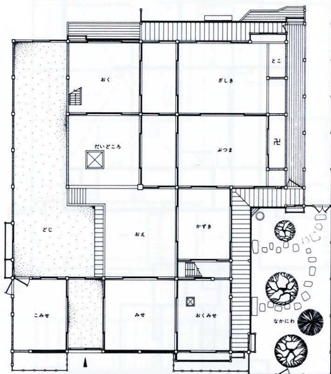
24-a 1階平面図
