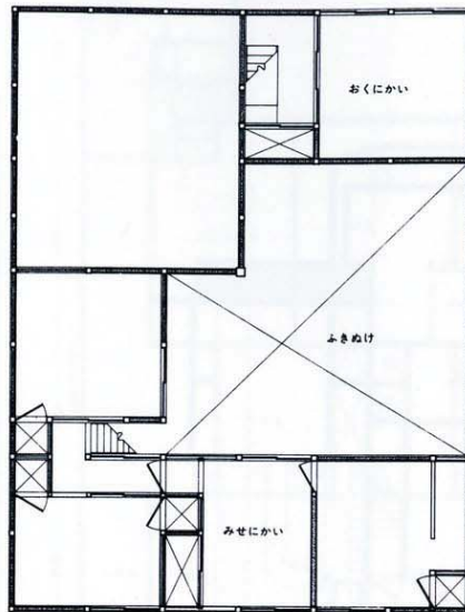
21-b 2階平面図
