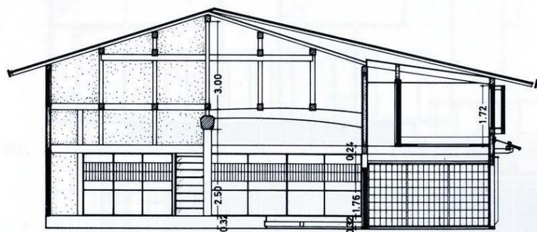
断面図
