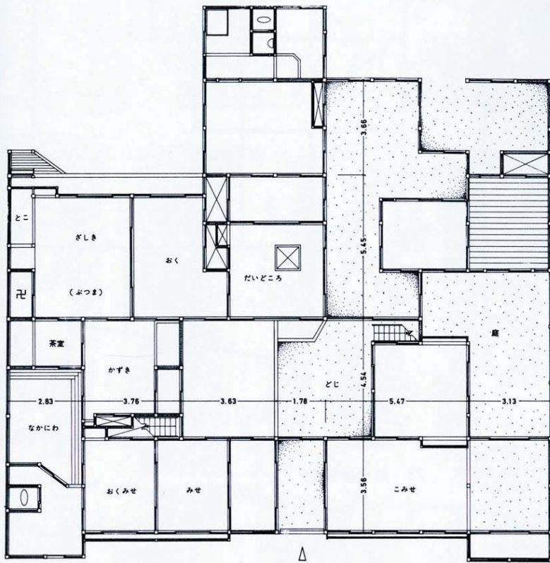
26-a | 1階平面図
