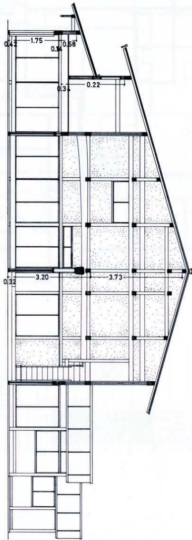
23-d 断面図
