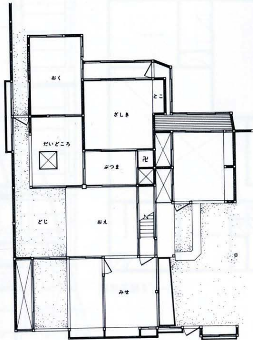
19-a 1階平面図
