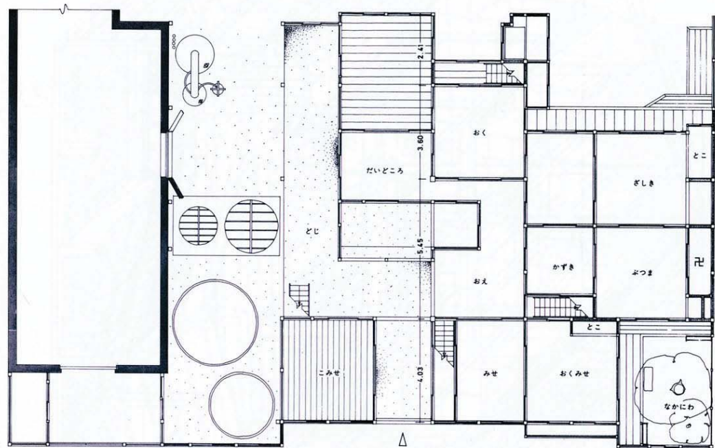
14-b 1階平面図
