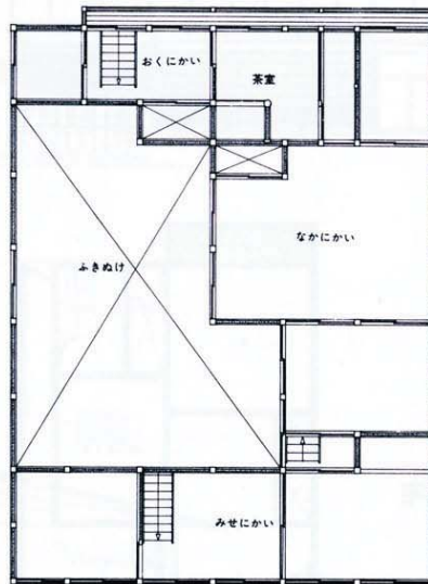
29-b 2階平面図
