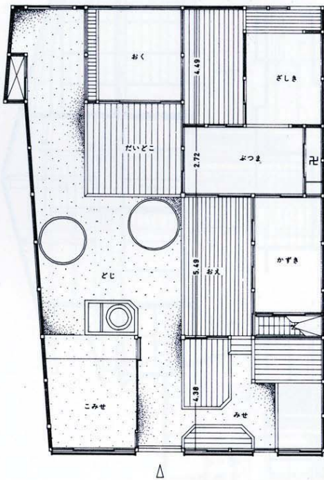
18-b 1階平面図
