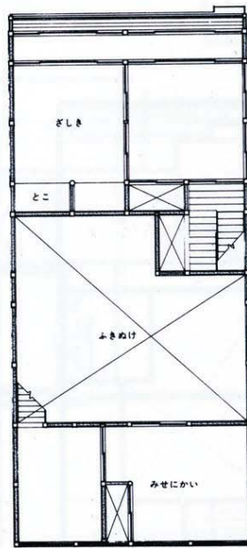
20-b 2階平面図
