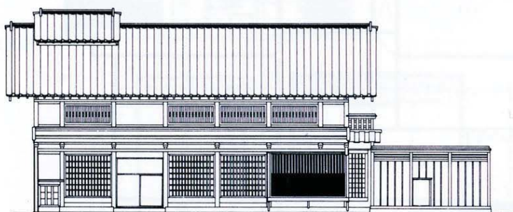
24-c 正面図
