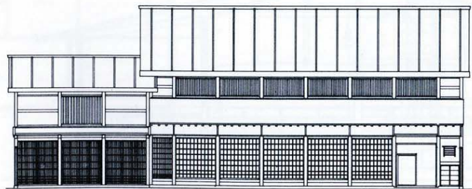
23-c 正面図
