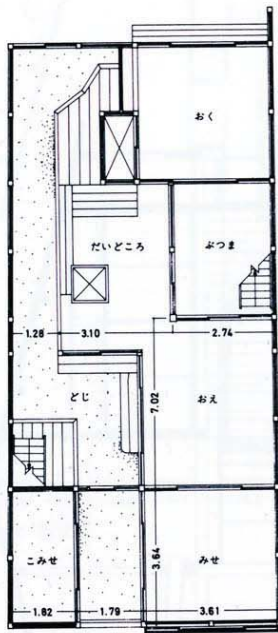
20-a 1階平面図
