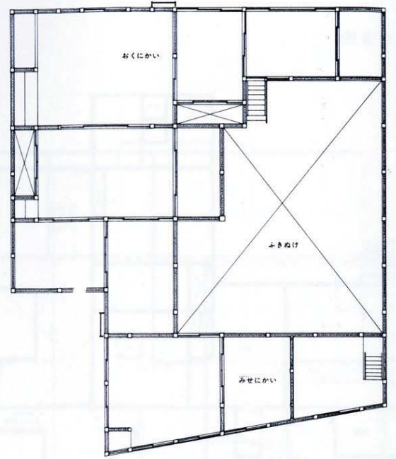
28-b 2階平面図
