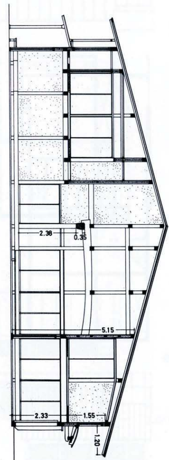
20-d 断面図
