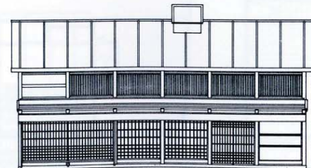
16-c 正面図
