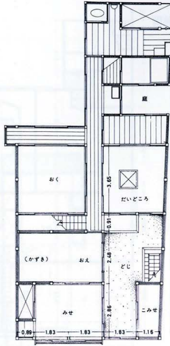
15-b 1階平面図
