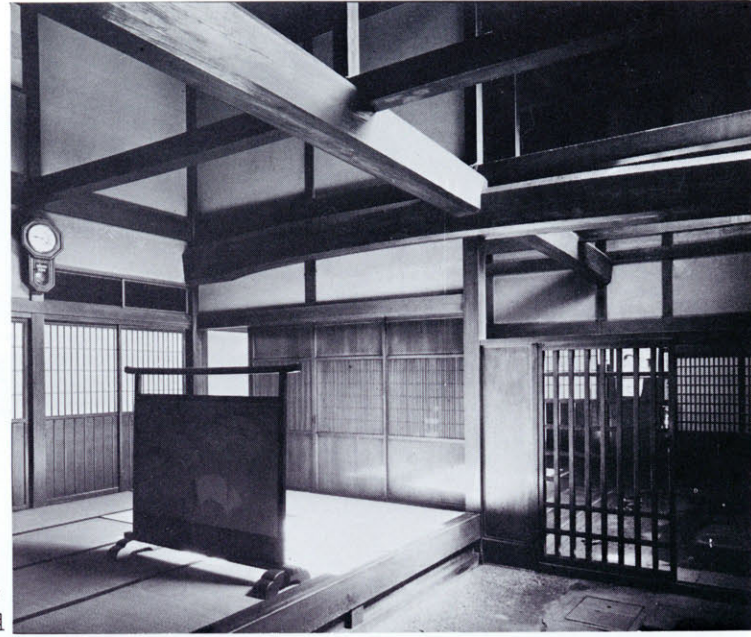
53-c おえ梁組
