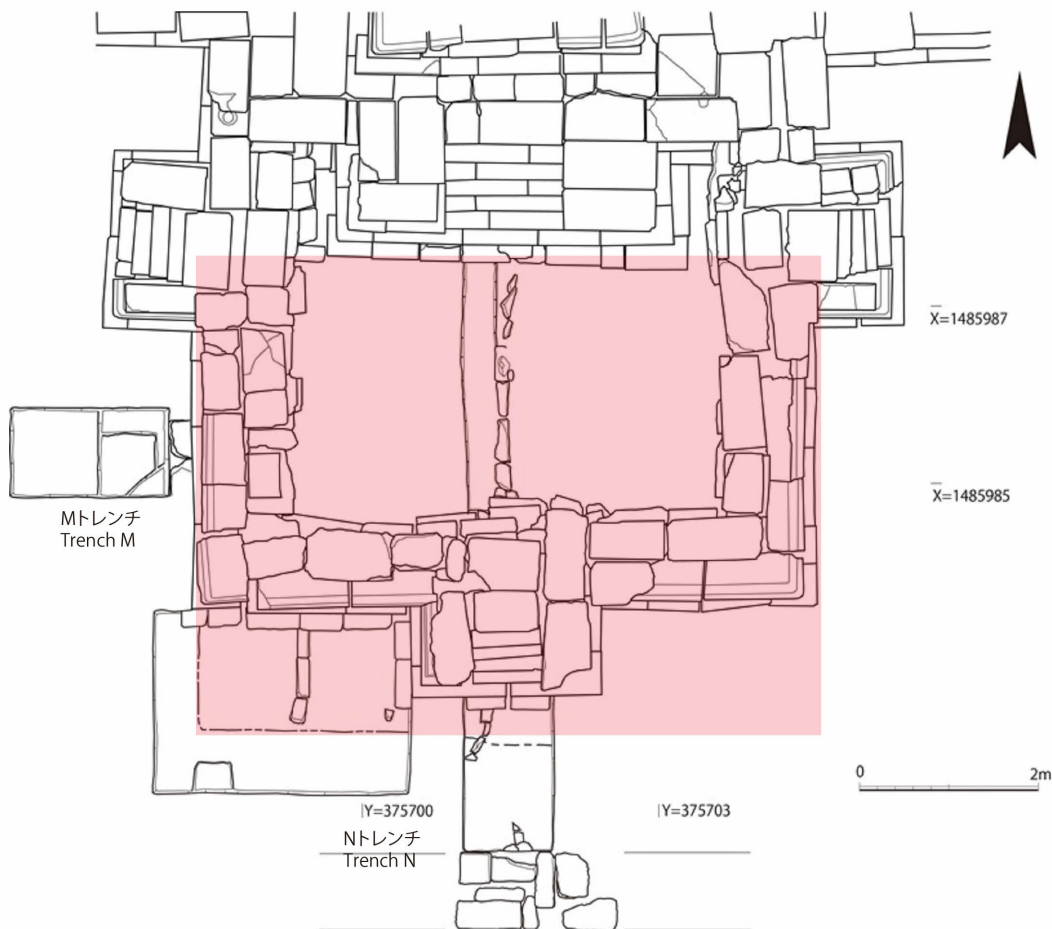
南祠堂の平面図と想定される「掘込地業」の範囲（ピンク色で示した部分）
