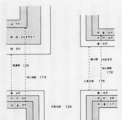
第8図 平安宮東南隅大路模式図 (「大内裏図考証」による)
