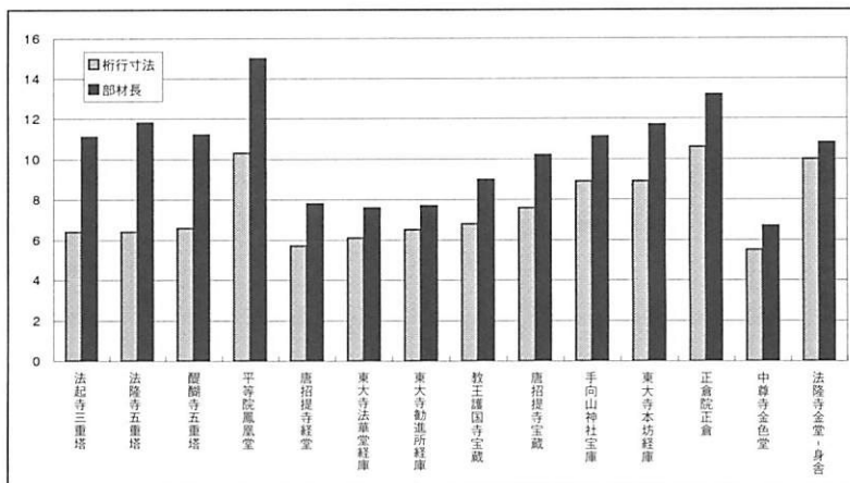
図2 建物規模と最大長材の長さ
