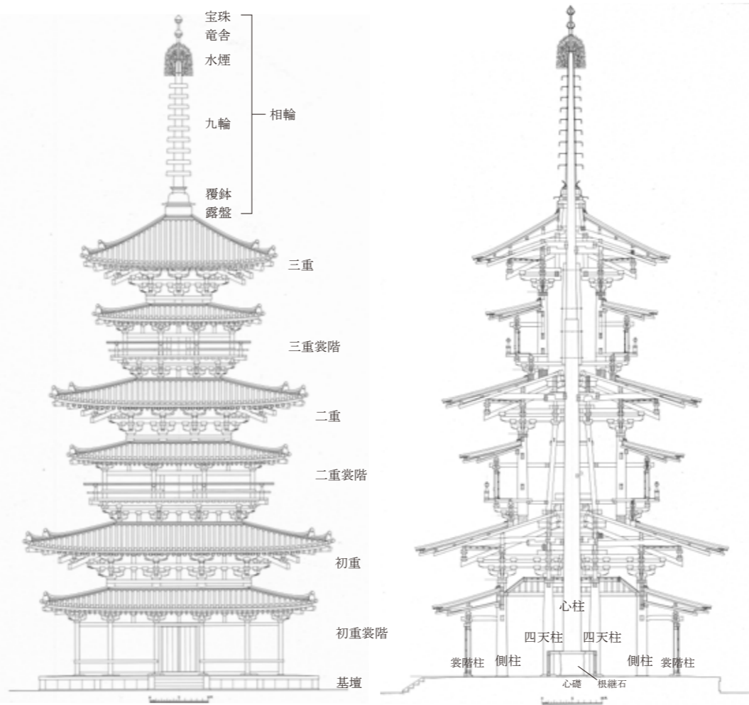
図3 東塔の各部名称
