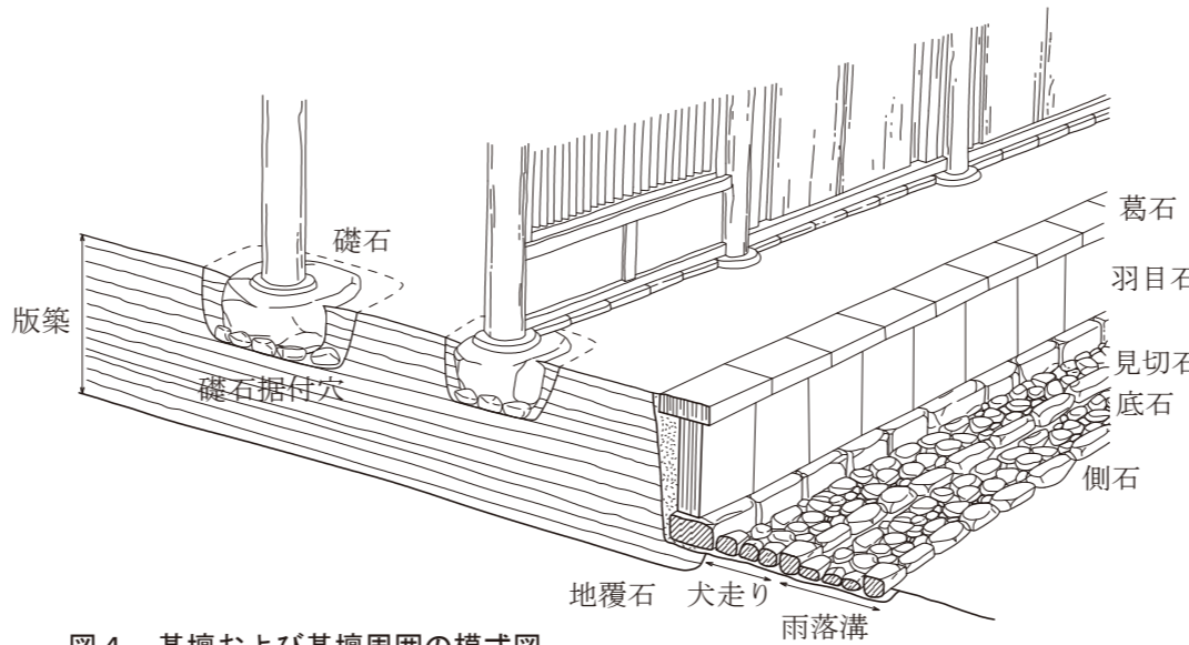
図4 基壇および基壇周囲の模式図
