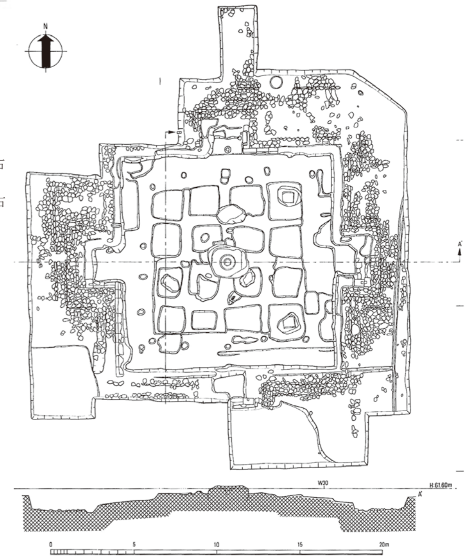
【参考】薬師寺西塔平面・断面図
