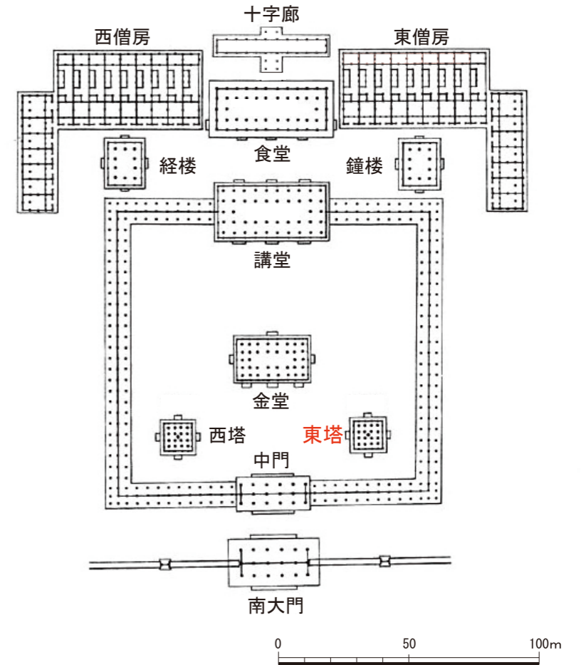
図6 薬師寺伽藍配置図
