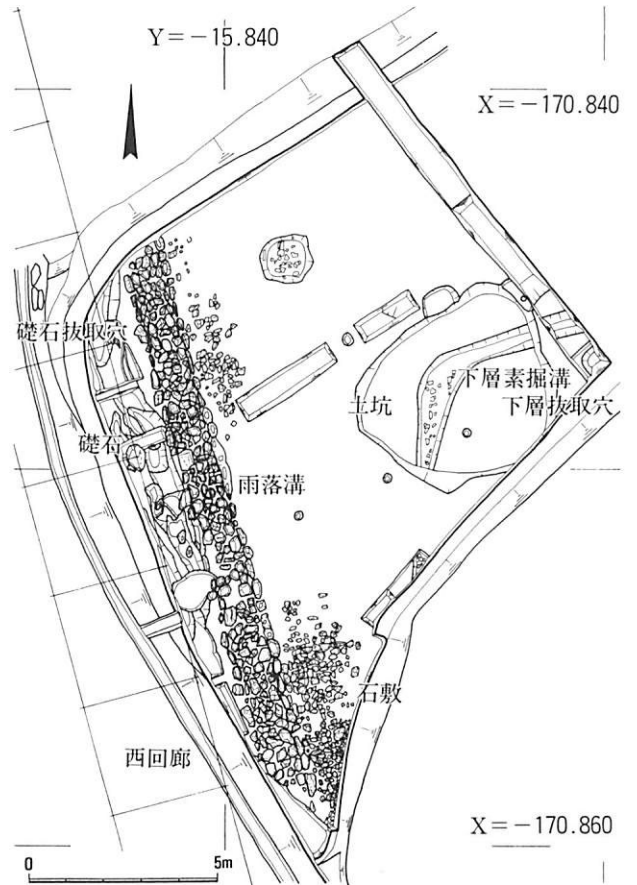
図66 坂田寺1996-1次調査遺構図 1:200
