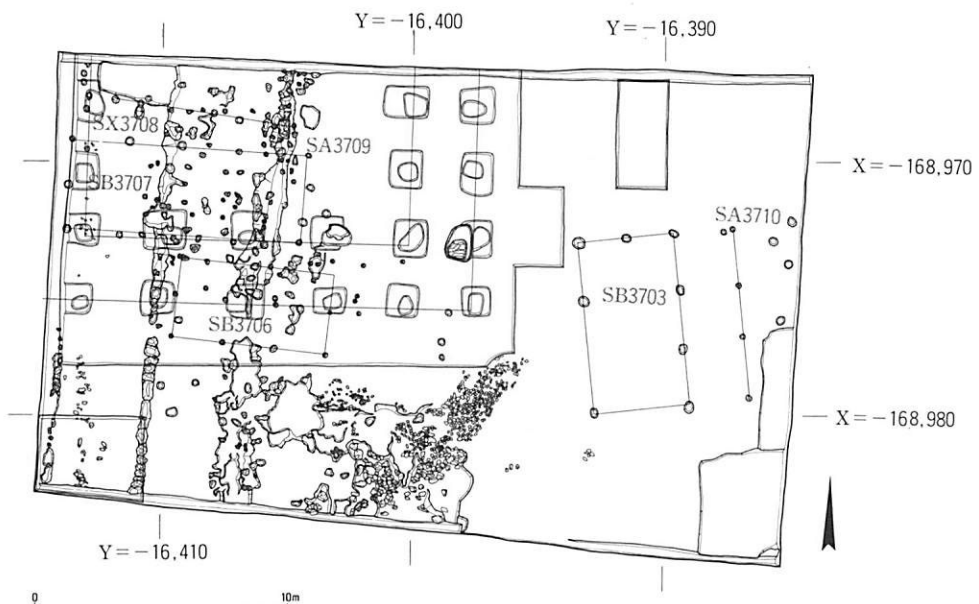
図38 水落遺跡第9次調査遺構図(上層) 1 : 300 色刷りは下層
