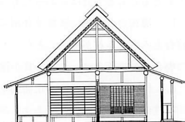
法蓮造農家断面図
