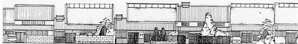
奈良法蓮の町並復原図
