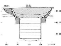
井戸 SE6 断面図 (1 : 160)
