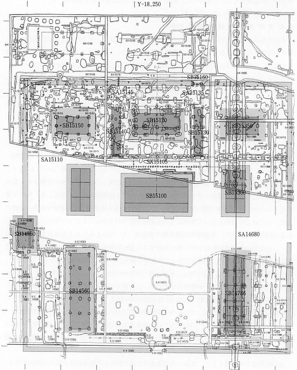
式部省調査遺構図(図A 上半第229・235次 下半第220次 1:600)
