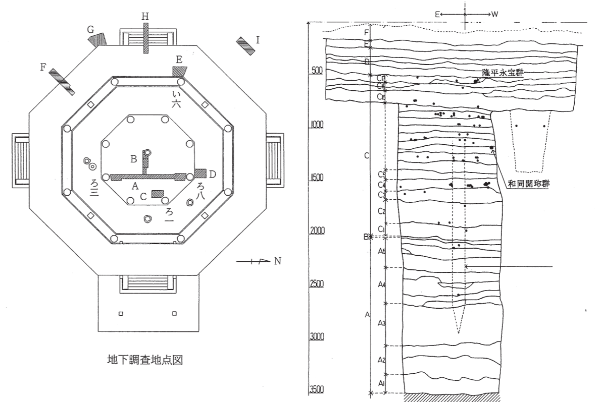
図4 西大寺東塔基壇の断面と銅銭出土位置 1:70 (奈文研 1982 『奈良国立文化財研究所年報 1982』)
