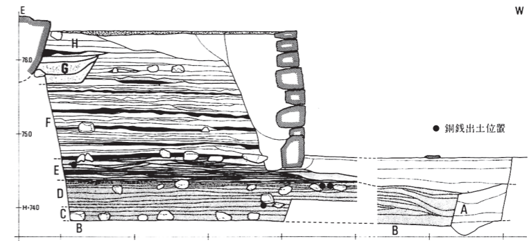
図4 西大寺東塔基壇の断面と銅銭出土位置 1:70 (奈文研 1982 『奈良国立文化財研究所年報 1982』)
