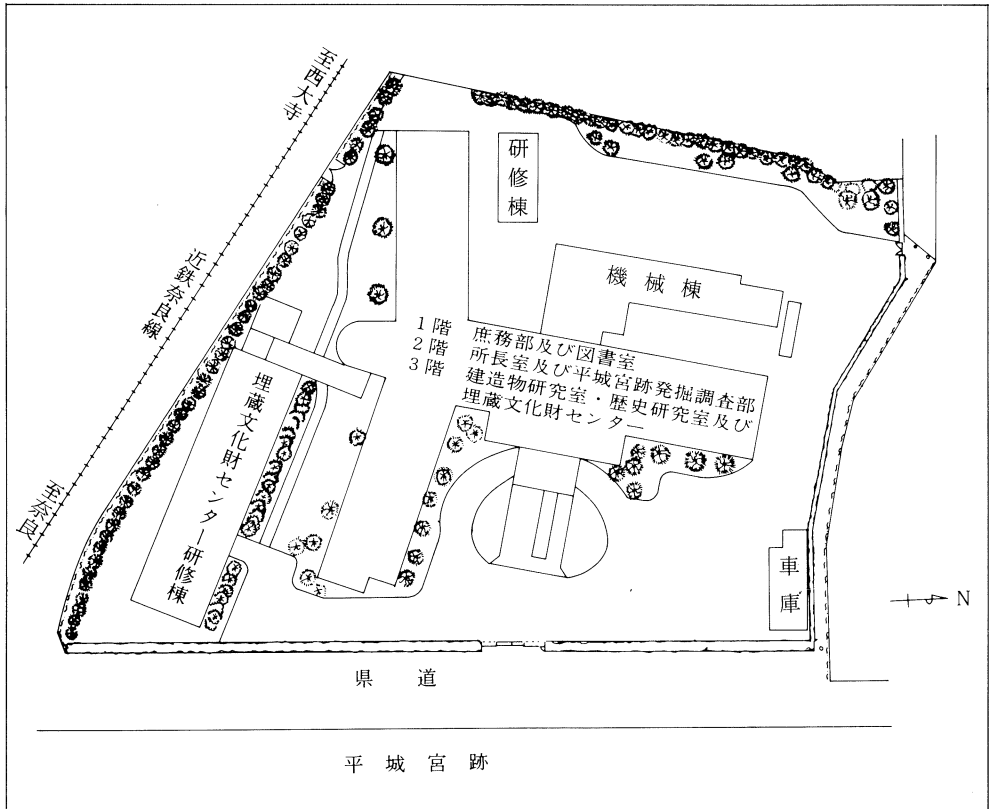
本館配置図
