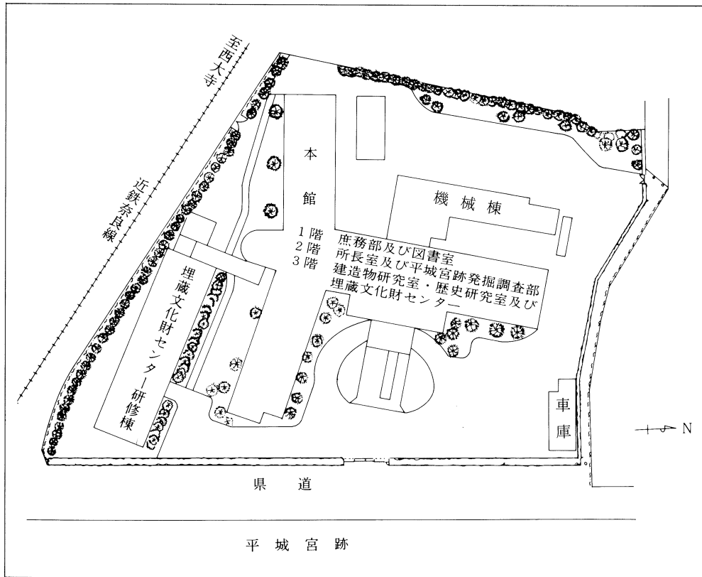
本館配置図
