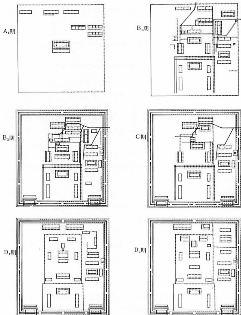
第3図 推定第2次内裏変遷図
