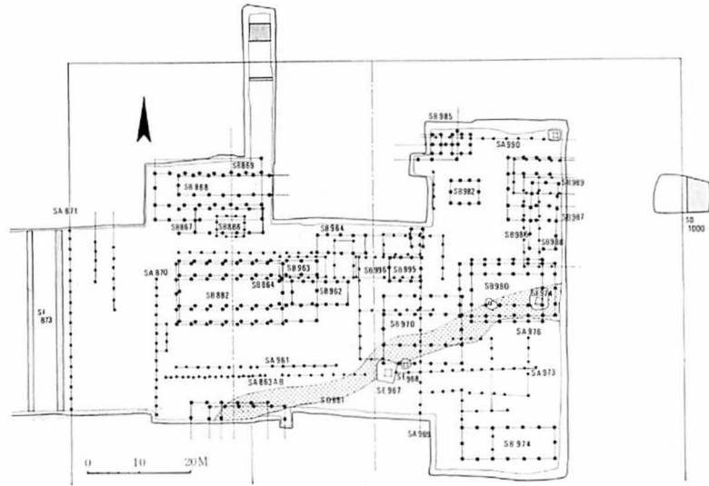
第7図 左京3条2坊15坪遺構配置図
