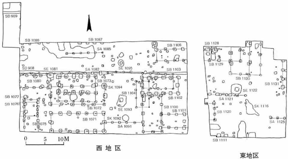
第9図 左京5条1坊4・5坪遺構実測図
