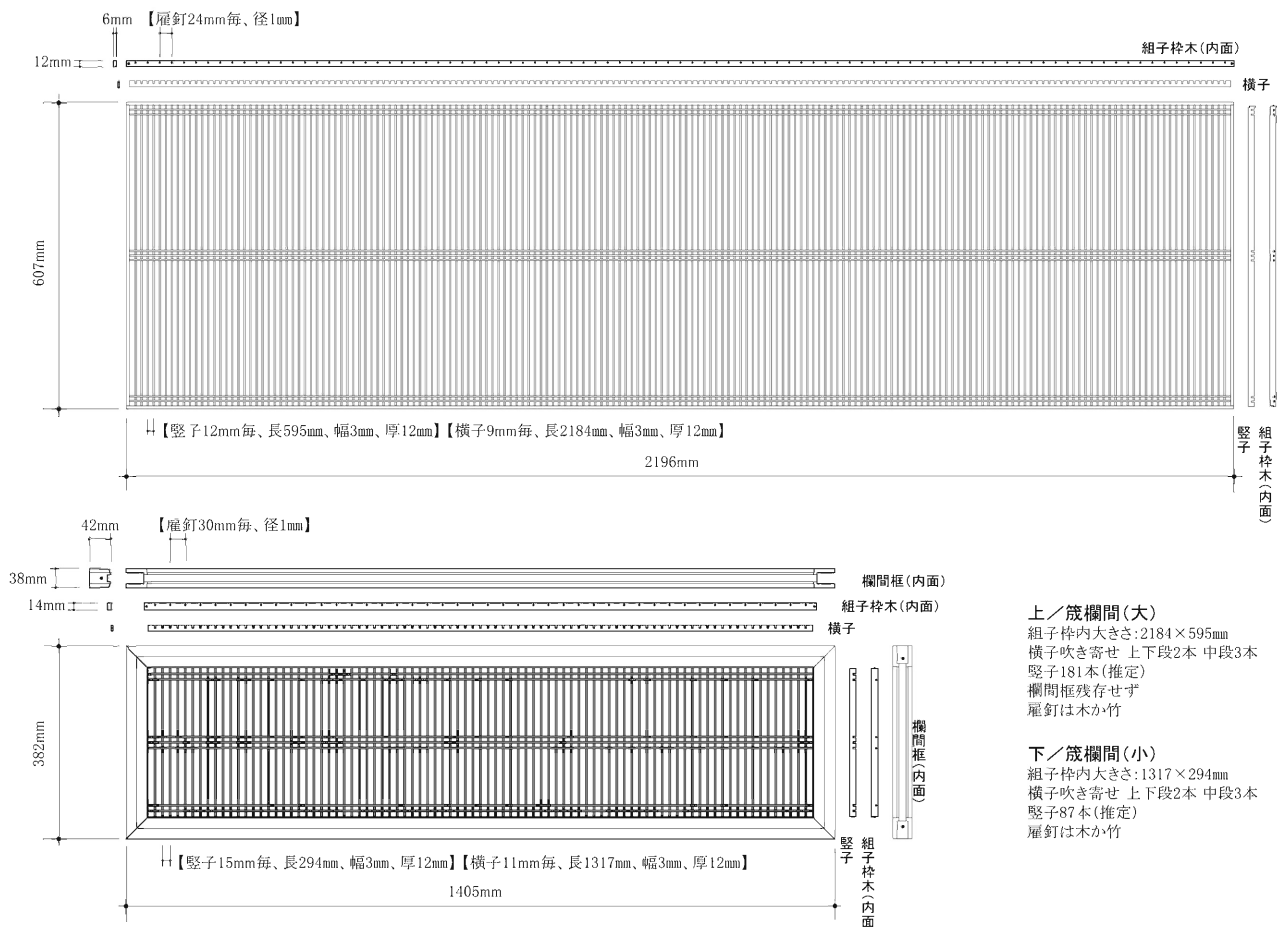
図13 茨木遺跡出土箄欄間 1:15
