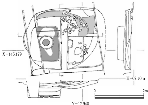
図 180 鑄造土坑 SX9220 平面図・断面図 1:80
