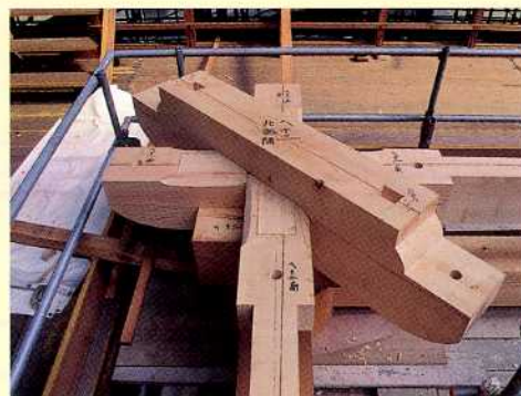
組物を組む (柱の上に部材を組みあげていきます)
