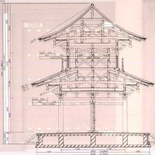
復原実施断面図
