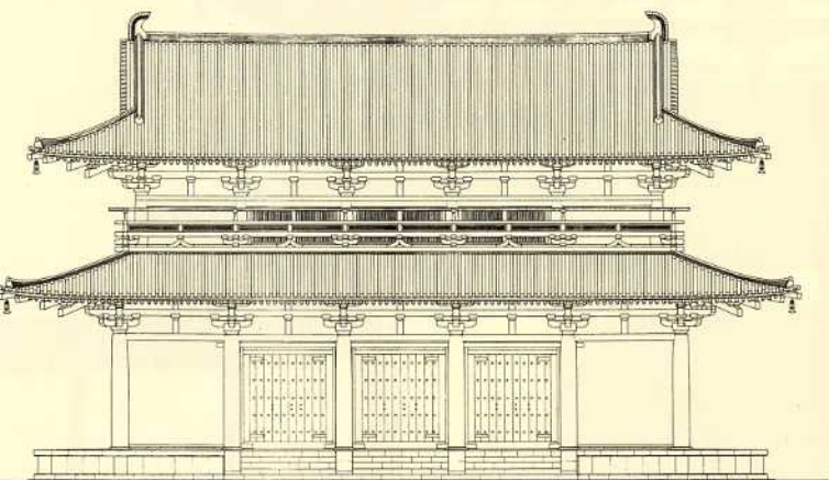
復原立面図
