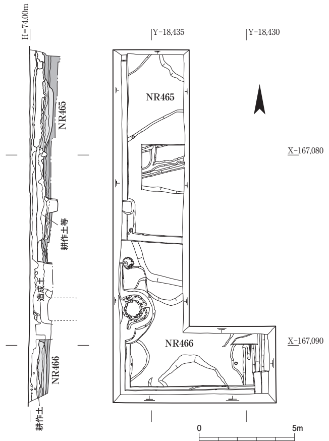
図150 第178-11次調査遺構図・土層図 1 : 200
