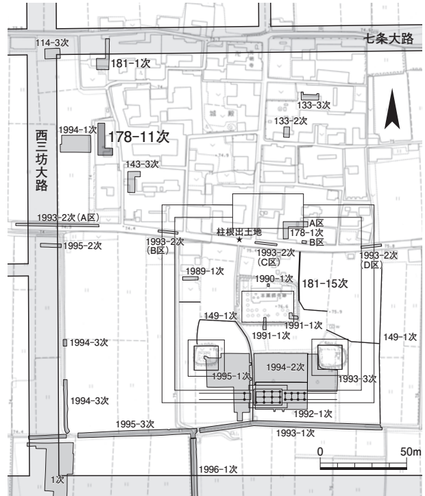
図149 第178-11次調査区位置図 1 : 3000
