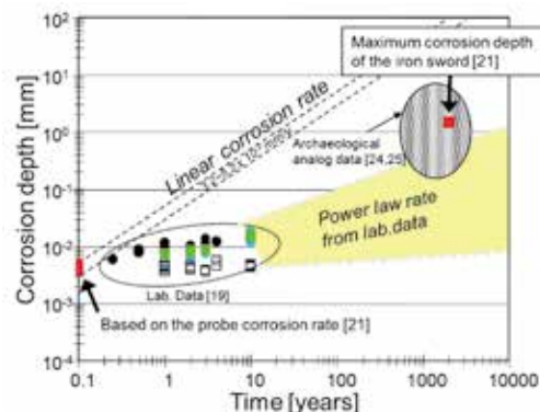
図12 : 腐食深さの経時変化の比較
