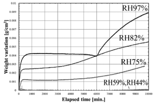
図4：1 mg/cm 2 試料の重量の変化
