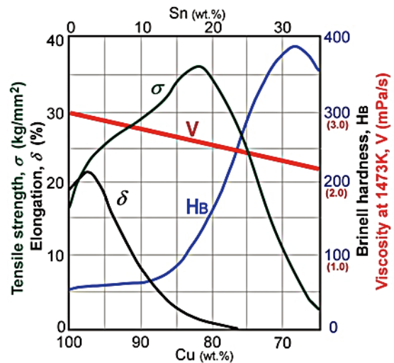
図6：銅—錫合金の物性と化学組成の相関 物性に関する数値はScott [5]を、粘度に関する数値はKozlov et al. [4].を参照した。
