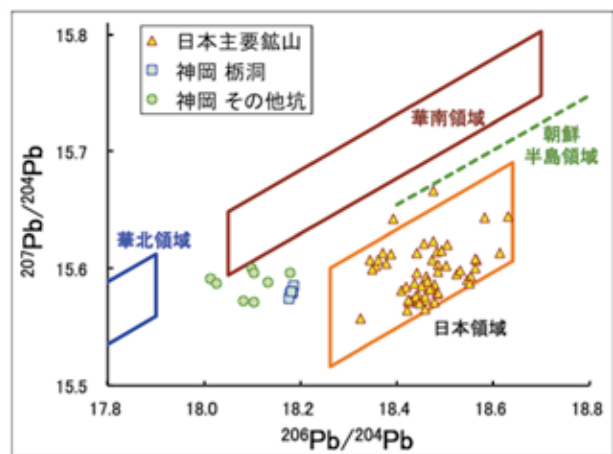
図5 鉛同位体比分布 (B式図)
