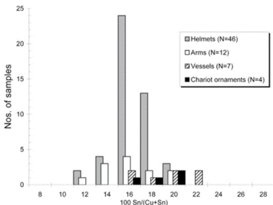
図5：EPMA法による各試料断面の平均化学組成銅—錫重量比（錫比）（ 100\text{Sn}/[\text{Cu}+\text{Sn}] ）の器種別頻度分布 Nは機種ごとの分析試料数を示す。（Iizuka & Uchida[1]）
