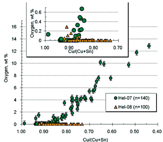
図4：HPKM1004 出土の青銅冑の化学組成分布 横軸は銅-錫重量比 ( \text{Cu}/[\text{Cu}+\text{Sn}] )、縦軸は酸素 (重量%)、n は EPMA による分析スポット数、上図は下図の一部を拡大したもの
