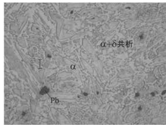
図2：Cu-23Sn-3Pb鑄造合金の組織
