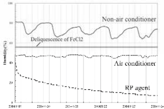
図 10：空調設備をとまなわない収蔵庫、空調設備で RH を制御した収蔵庫、ガスバリアフィルムと除湿剤を用いた環境管理での相対湿度の比較
