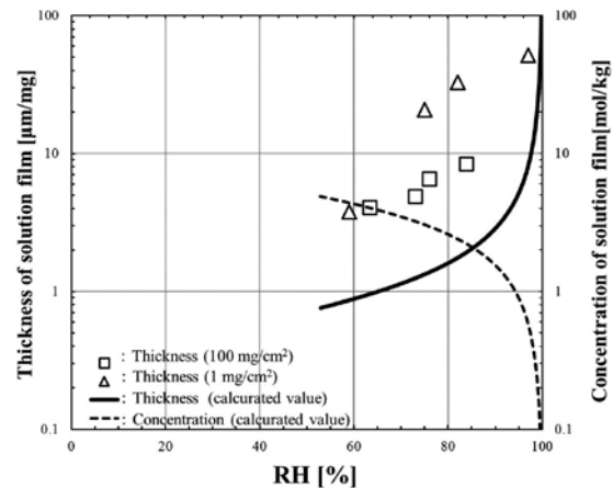
図5：RHと水膜厚さ、水膜のFeCl 2 濃度の関係
