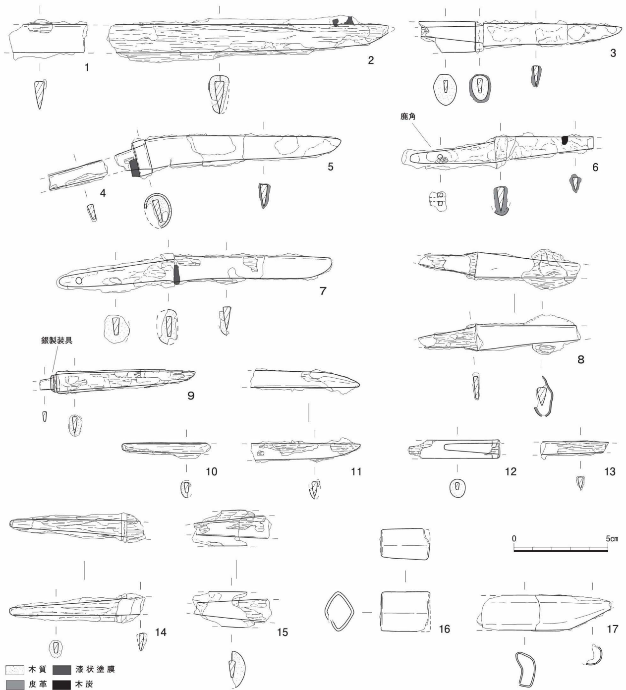
図16 刀子実測図 1:2
