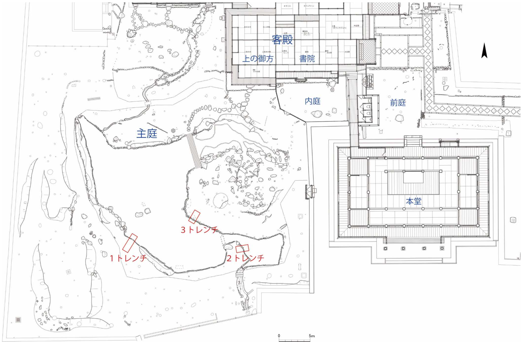
図1 平城第618次調査 トレンチ配置図 1:300
