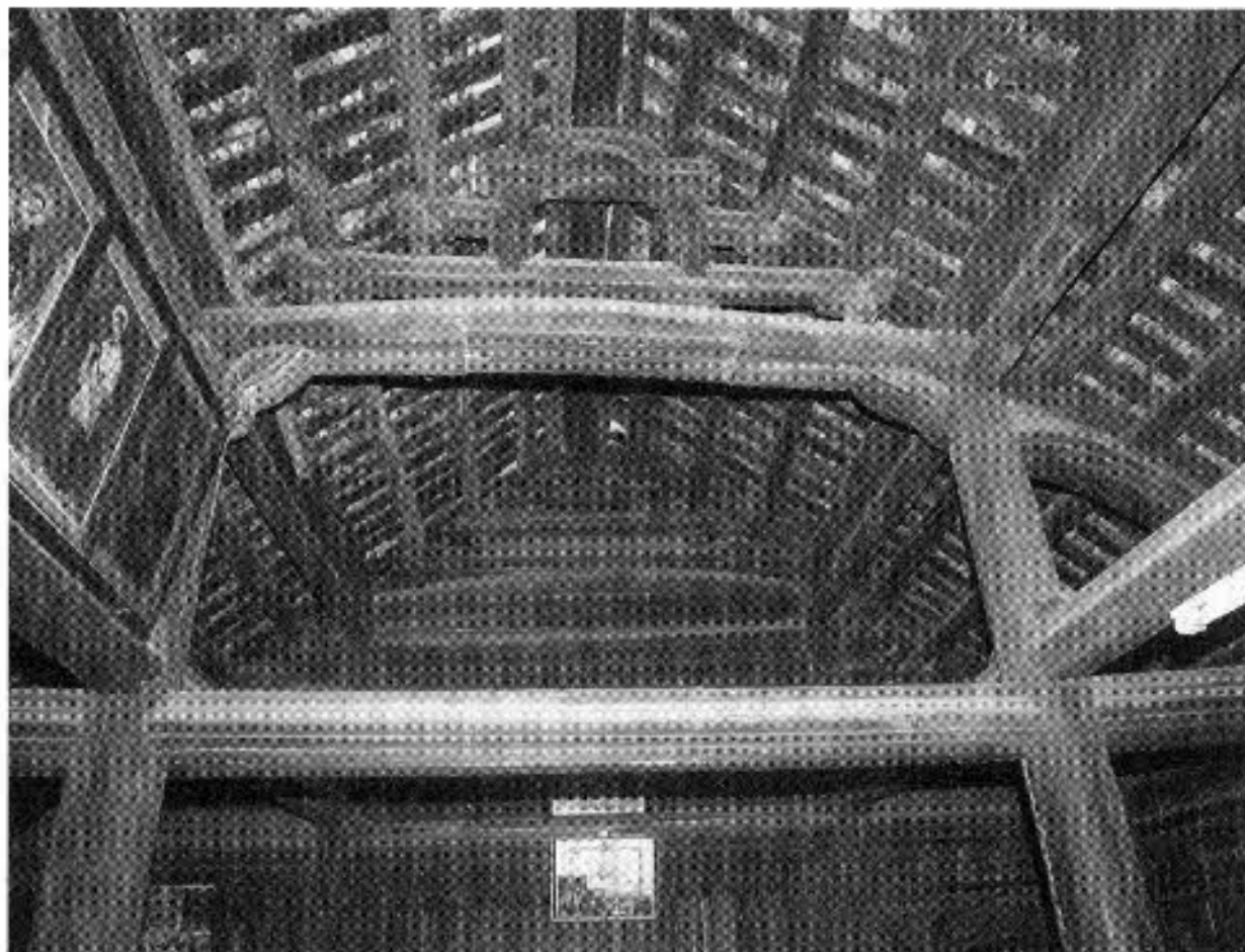
図27 モンフーⅡ-55宅の主屋内部
