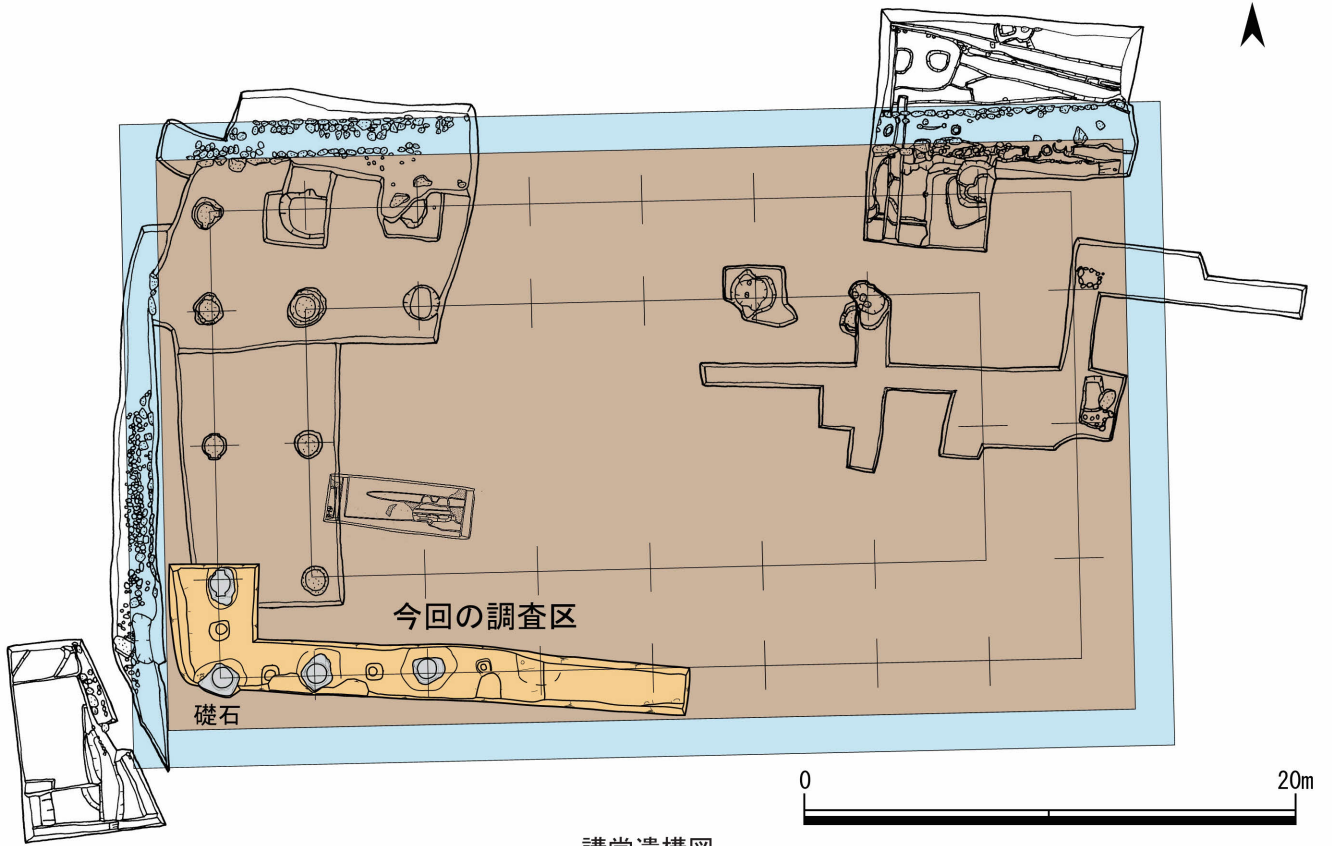
講堂遺構図
