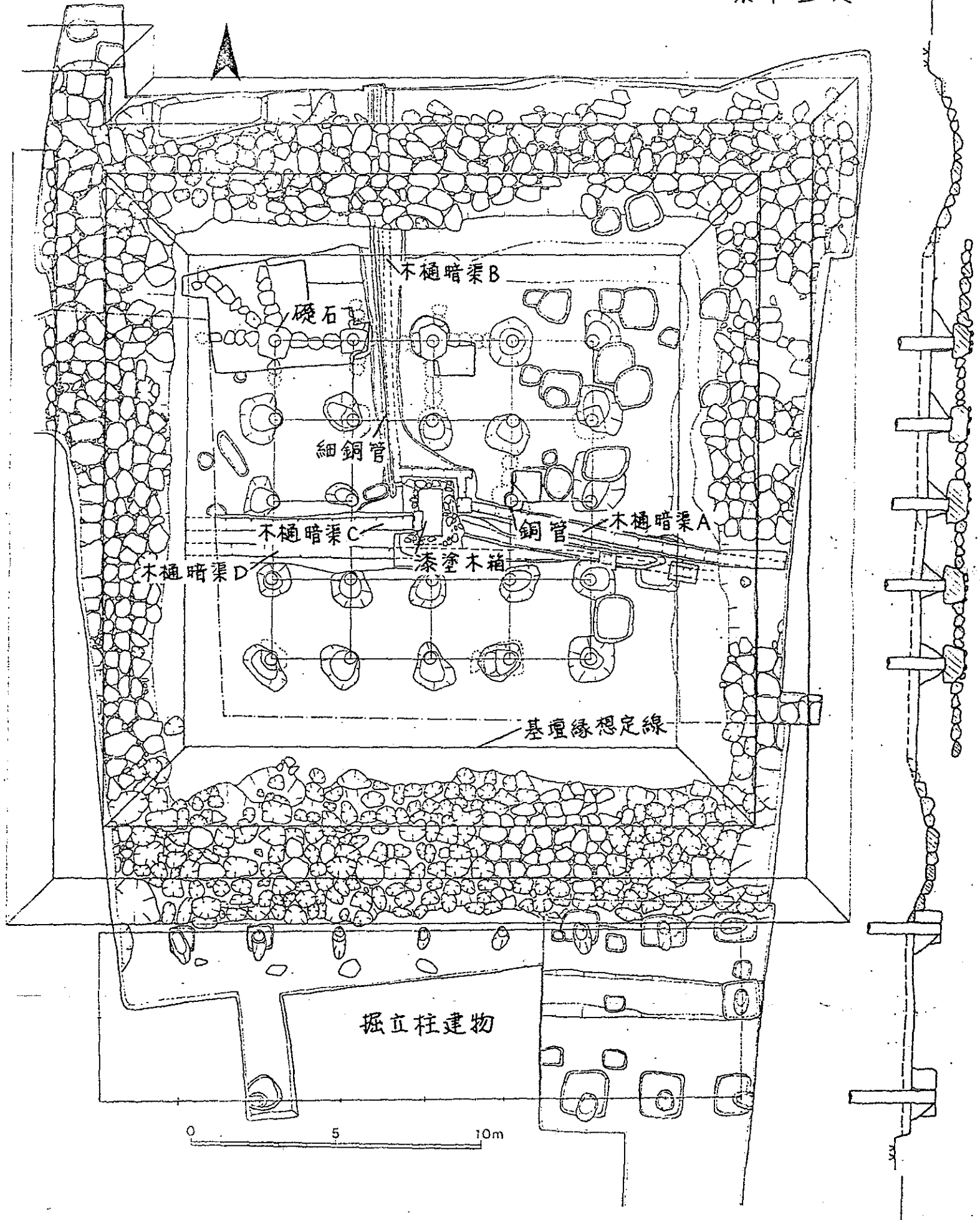
飛鳥水落遺跡遺構圖
