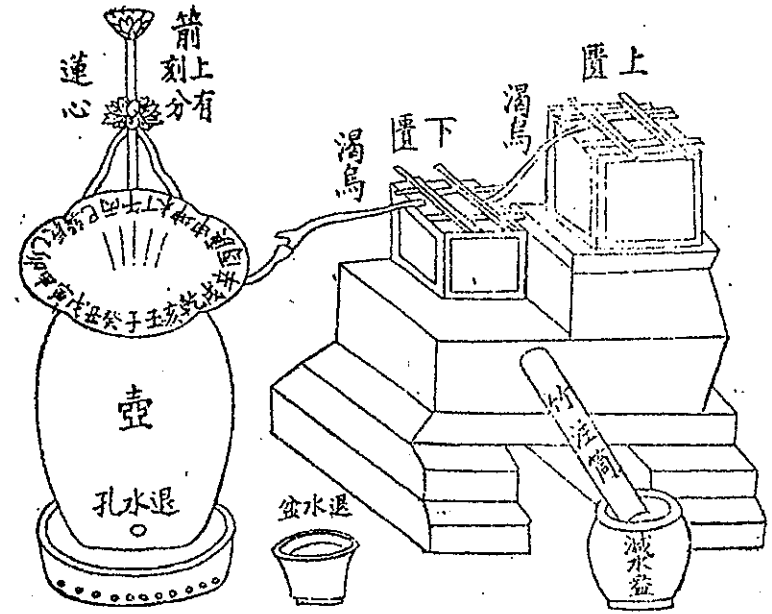
图 9-19 宋燕肃漏刻图，采自《古今图书集成·历法典·第九十九卷》。图中竹注筒位置有误，上端应上接下甌，此图却绘于底座边上了。
