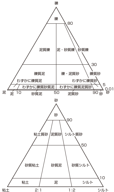
図1 粒度組成に基づく土質分類
