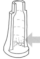
6284 Eb(1) 丸瓦部凹面から接合部にかけてのこる指頭ないし先端円形工具の圧痕(1:5)
