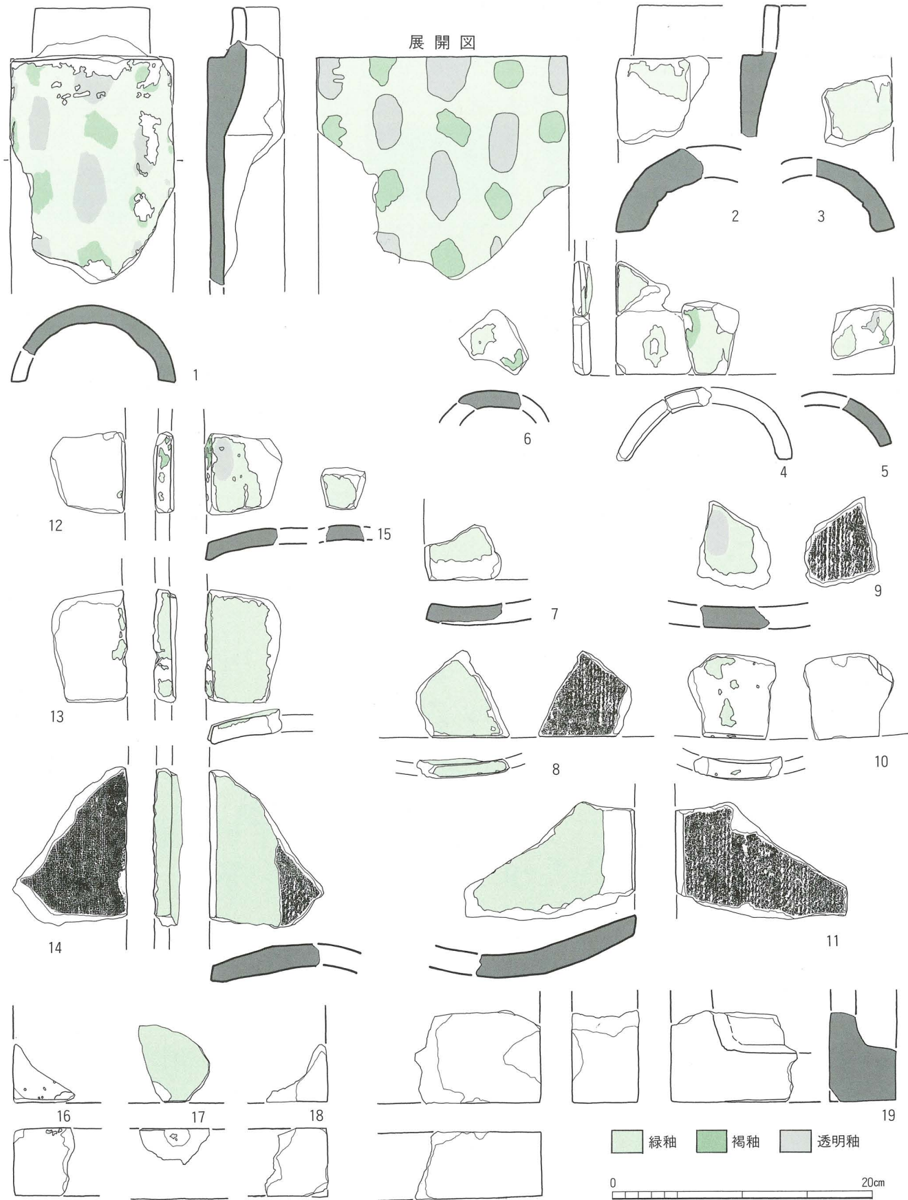
1~6 丸瓦 7~11 平瓦 12~15 鬩斗瓦 16~19 塼 1:4
