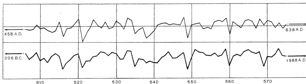
Fig. 89 ヒノキの暦年標準パターングラフ(下)と折敷(杉材)の年輪変動パターングラフ(上)
