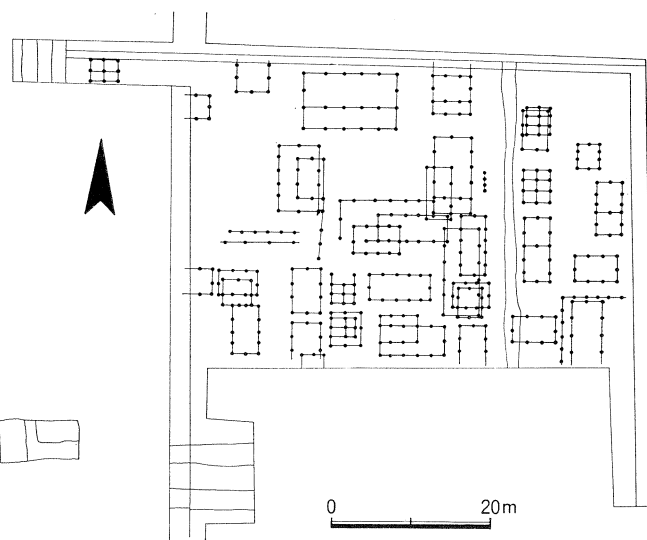
Fig. 82 左京六条二坊十四坪
