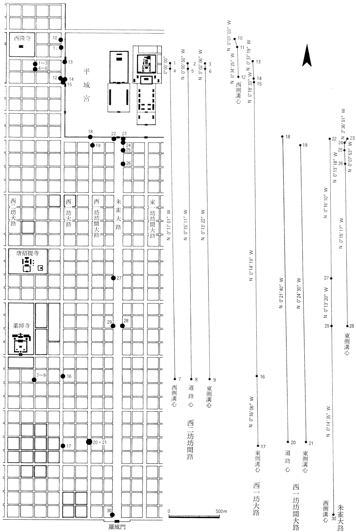
Fig. 69 平城京右京域の条坊道路の偏度 (図中の No. は Tab.20 と対応)
