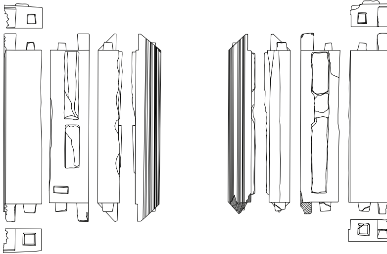
Fig.29 西面扉・垂直杵部材
