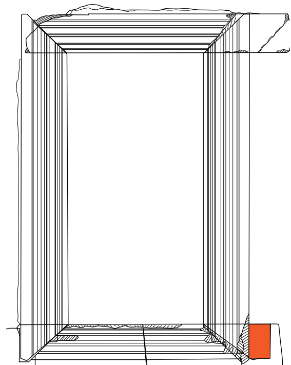
Fig.18 西面扉枠実測図 (赤色部分は接合時の固定が完全ではない箇所)
