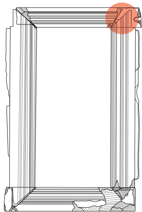
Fig.18 西面扉枠実測図 (赤色部分は接合時の固定が完全ではない箇所)
