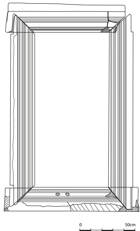
Fig.17 東面扉枠実測図
