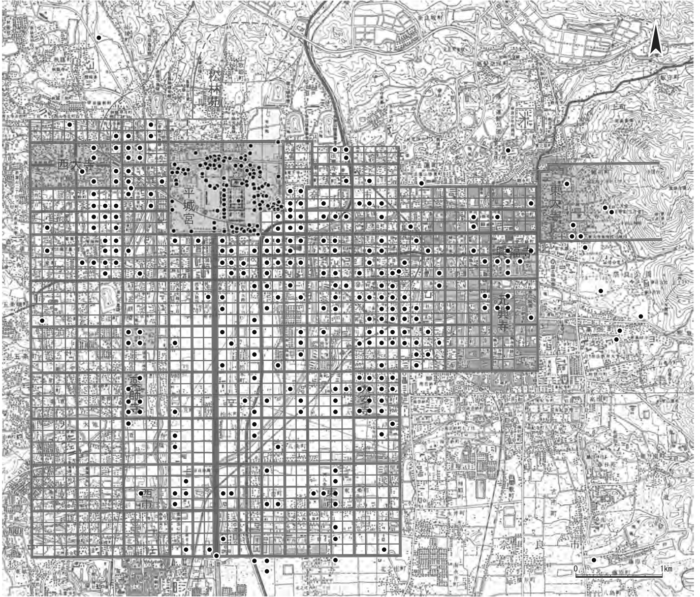
图 平城京墨書土器・刻書土器等出土地 1 : 45000
