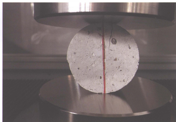
写2 割裂試験
